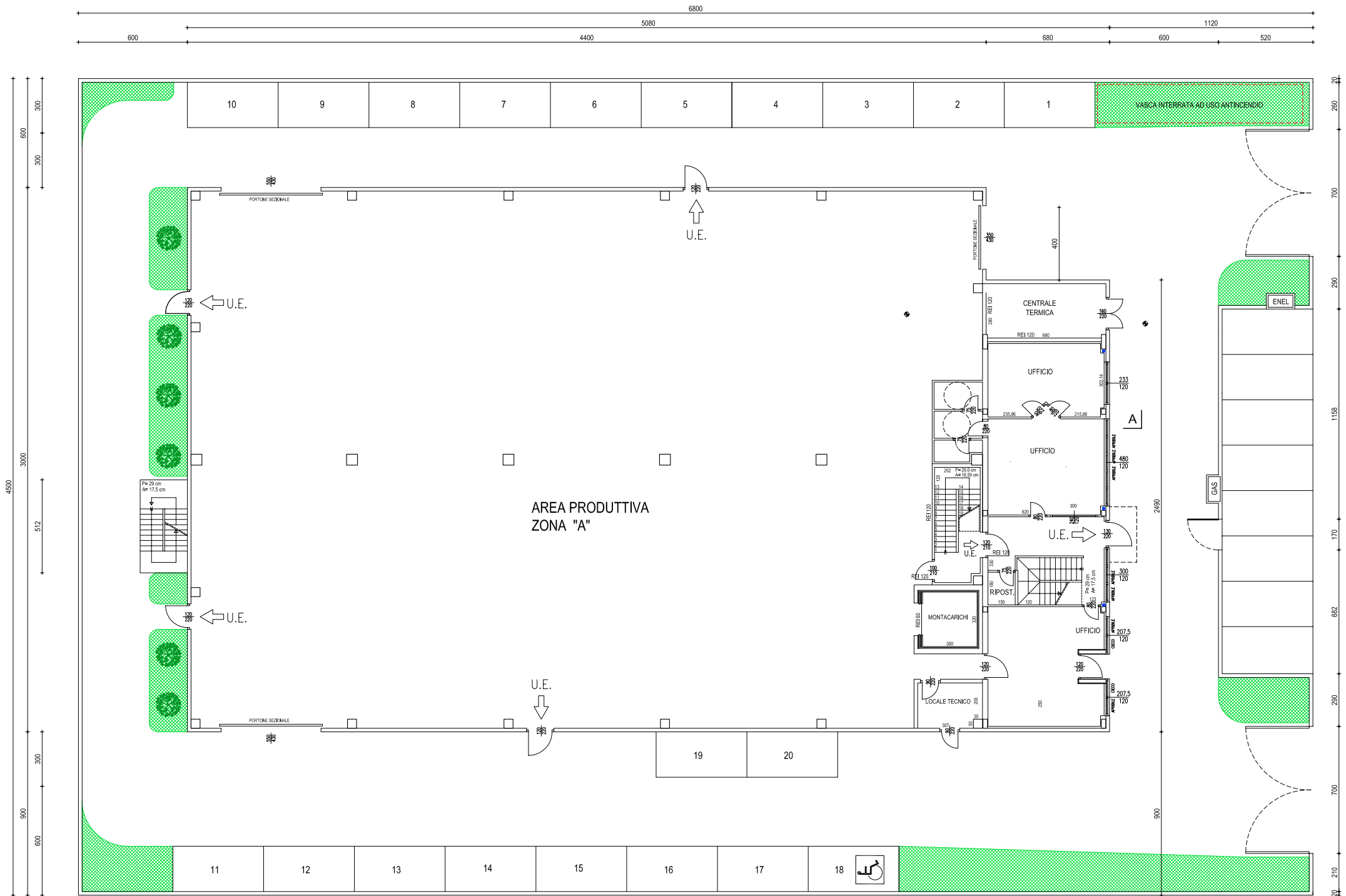
PLANIMETRIA GENERALE
